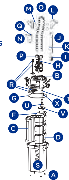
Fluval 206
