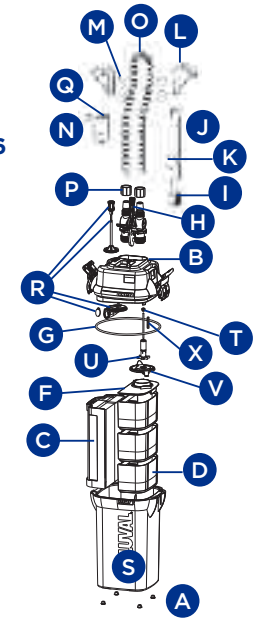
Fluval 206
